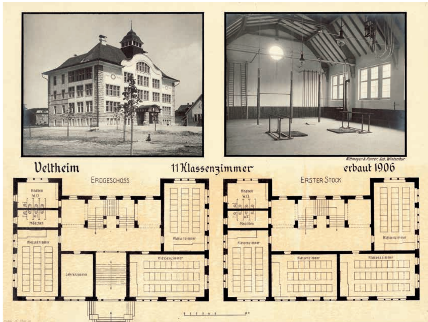
Rittmeyer & Furrer, Primarschule in Velt- heim ZH, erbaut 1906. Abbildungsnachweis: Staatsarchiv Zürich: Plan D 2334.16
